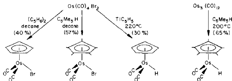
Scheme 22.
