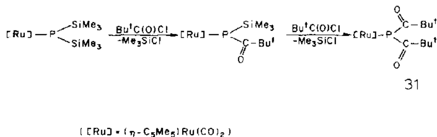
Scheme 18.
