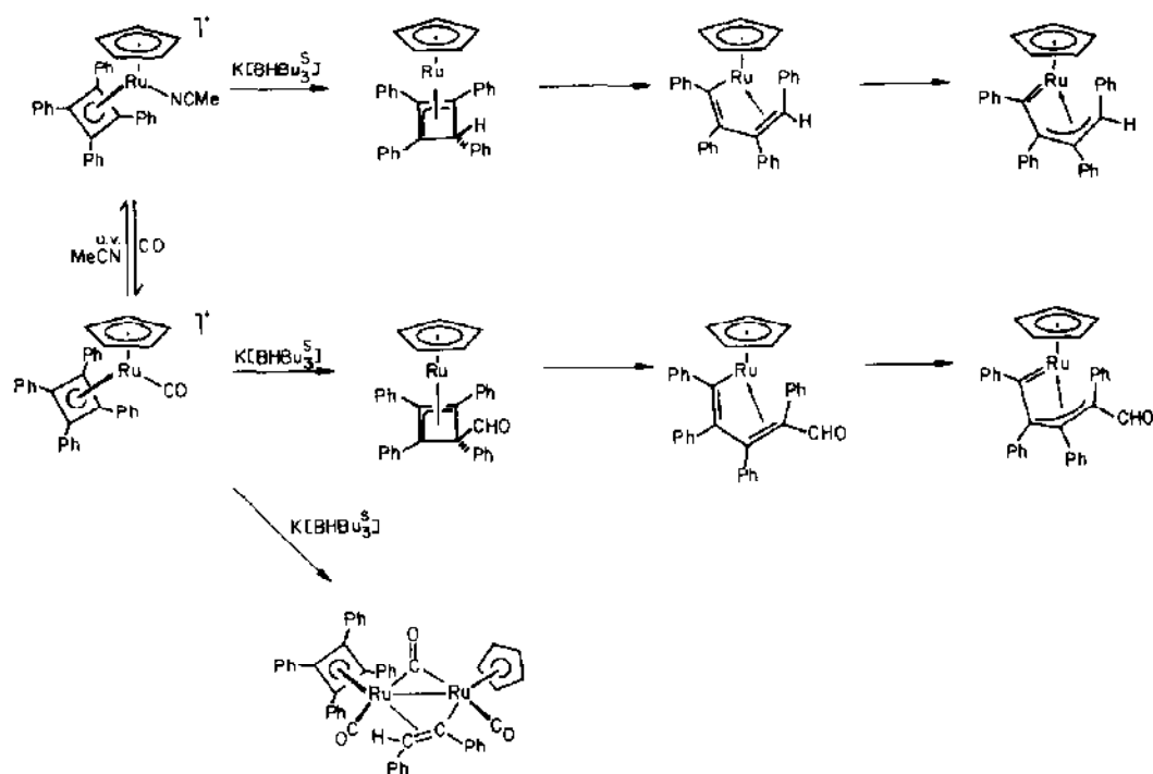
Scheme 45.
