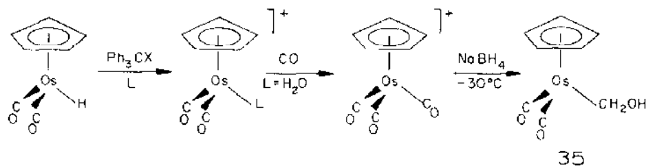
Scheme 23.
