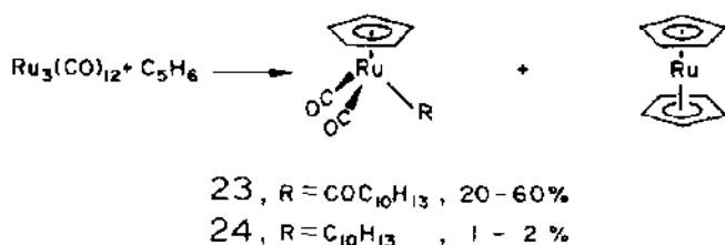
Scheme 14.
