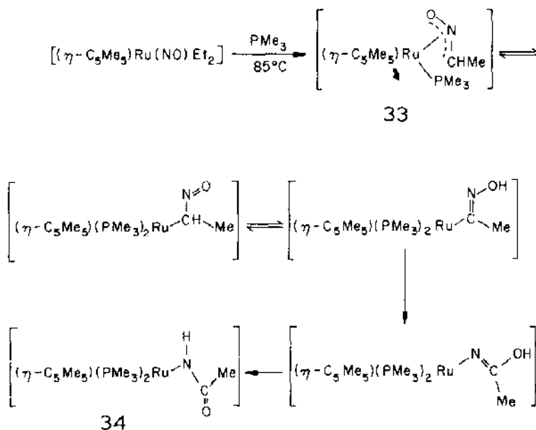
Scheme 21.
