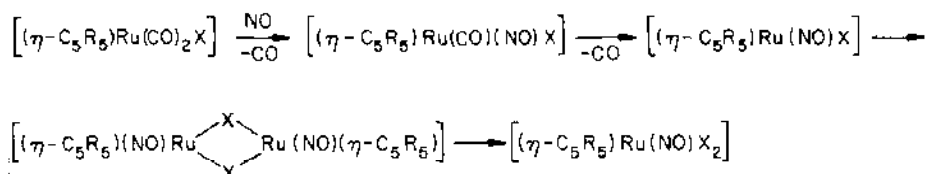
Scheme 19.
